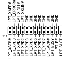
LPT
