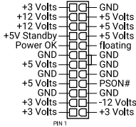
C ATX_PWR
